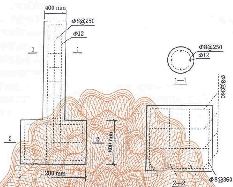
图 G.2 GPS 观测墩结构设计剖面图
