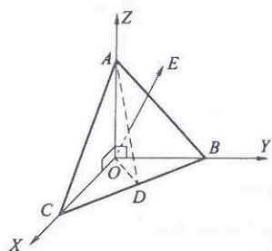
图 F.1 三面角反射器几何结构图
