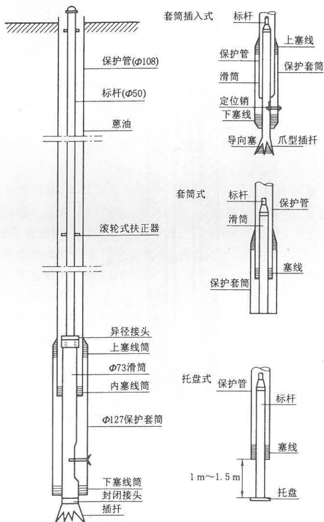
图 H.4 分层标标底结构示意图
