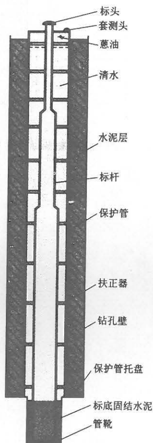
图 H.1 基岩标标型结构参考图
