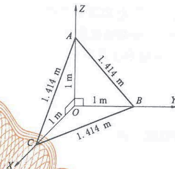
图 F.2 直角边长为 1 m 的三面角反射器几何结构
