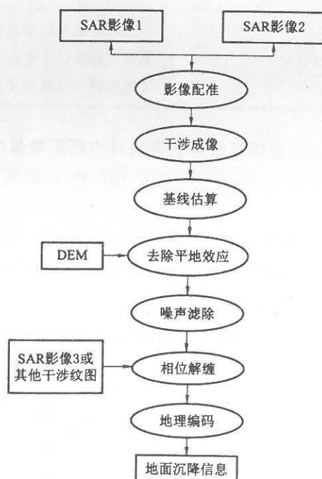
图 D.1 数据处理基本流程图
